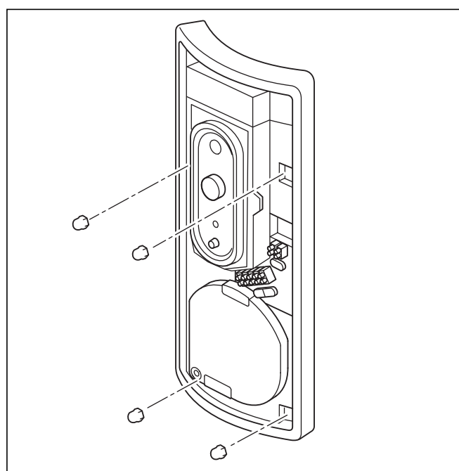
Рис. 7.15 Демонтаж электрокоробки
